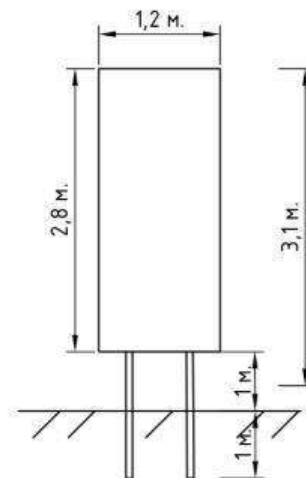
Макет двусторонней отдельностоящей рекламной конструкции
